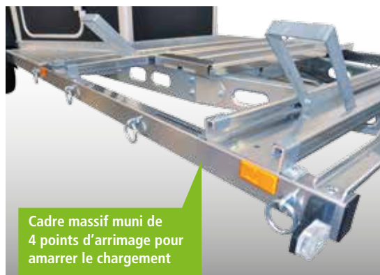
Porte-calèche Zephir® avec carrosserie tout polystère
